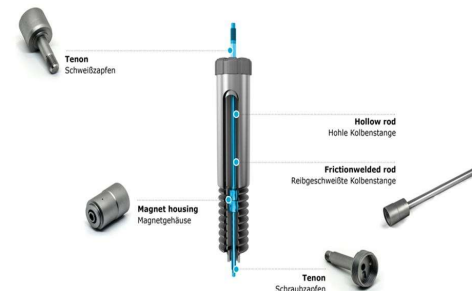
.... Shocks Absorber • Stoßdämpfer
